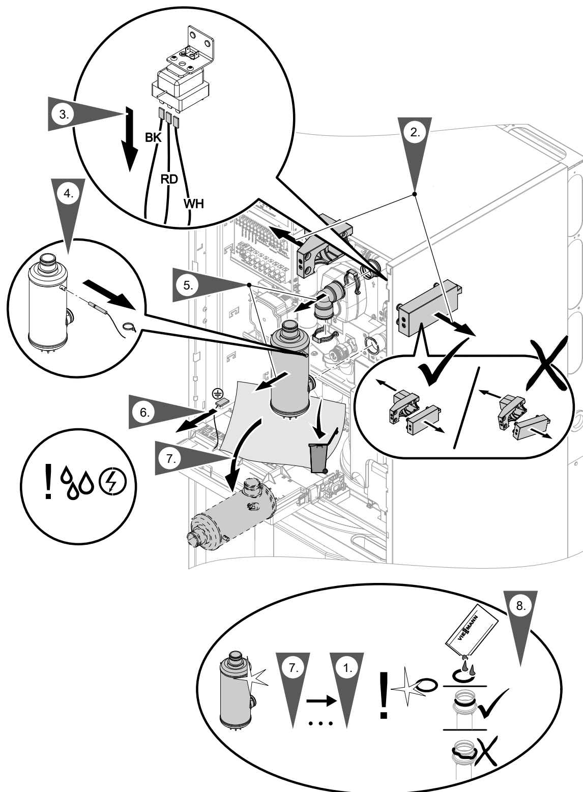
Rys. 88 Przestrzegać oznakowania kolorami żył podłączonych do zabezpieczającego ogranicznika temperatury (wg IEC 60757):
