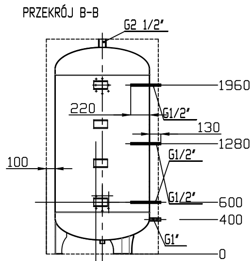
Bufor 2000 L DIS 2000
