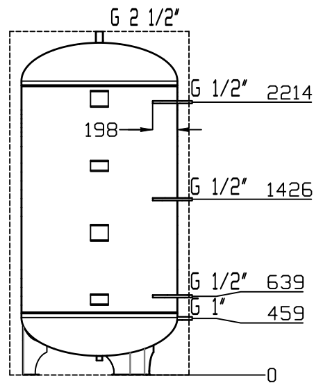
PRZEKRÓJ B-B
