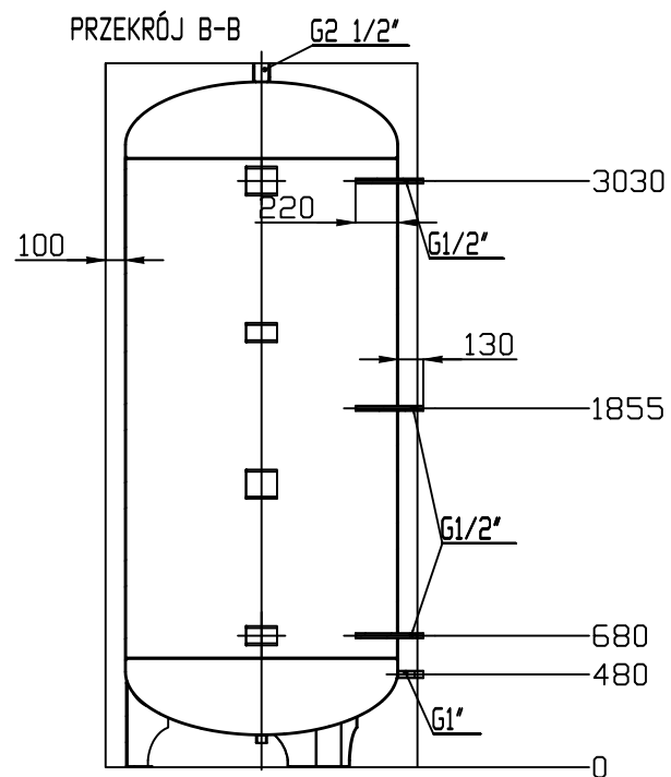
Bufor 5000 L DIS 5000
