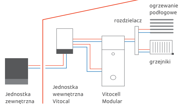
Vitocell Modular - pomyślany dla potrzeb pomp ciepła Vitocal
