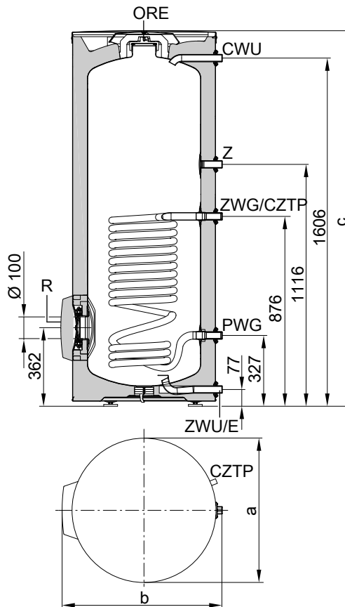
Wymiary typu EVIB-A, pojemność 300 l
